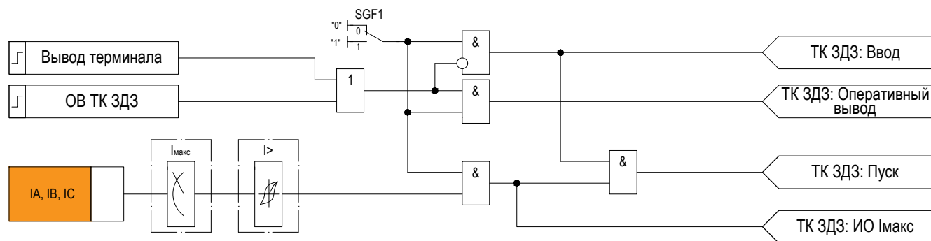
Рисунок 2.25 – Функциональная схема «ТК 3Д3»
