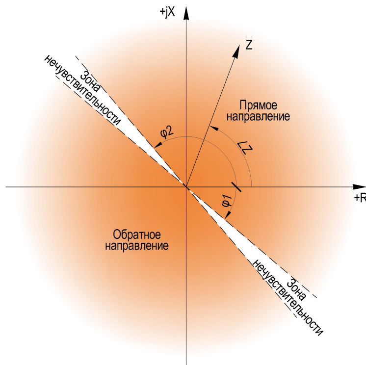
Рисунок 2.4 – Характеристика ОН
